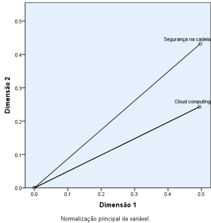
Ilustração 47 – Representação de “Segurança na cadeia de fornecimento” e “Cloud computing” nas componentes principais (loadings)
